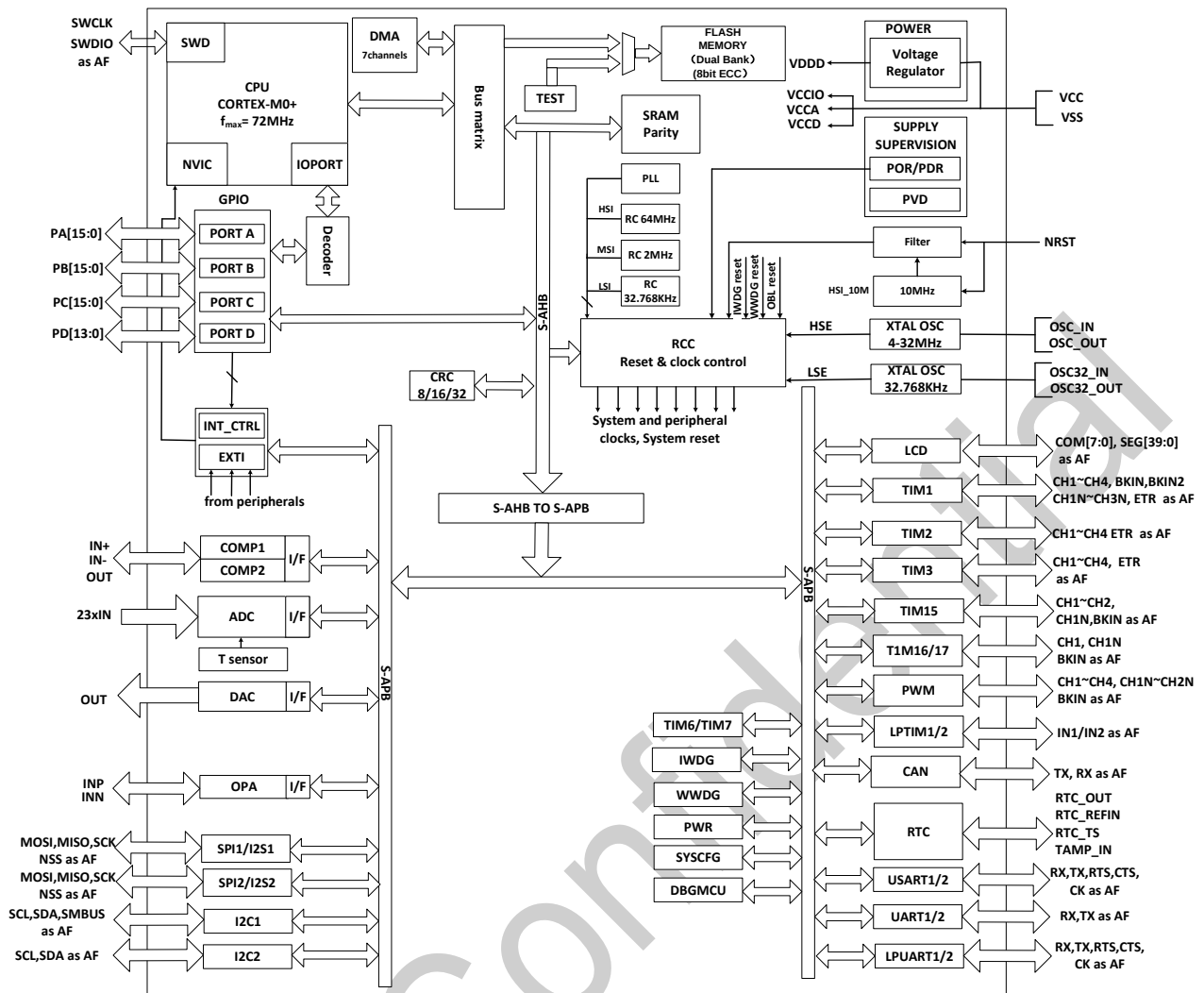
图 1-1 功能模块
