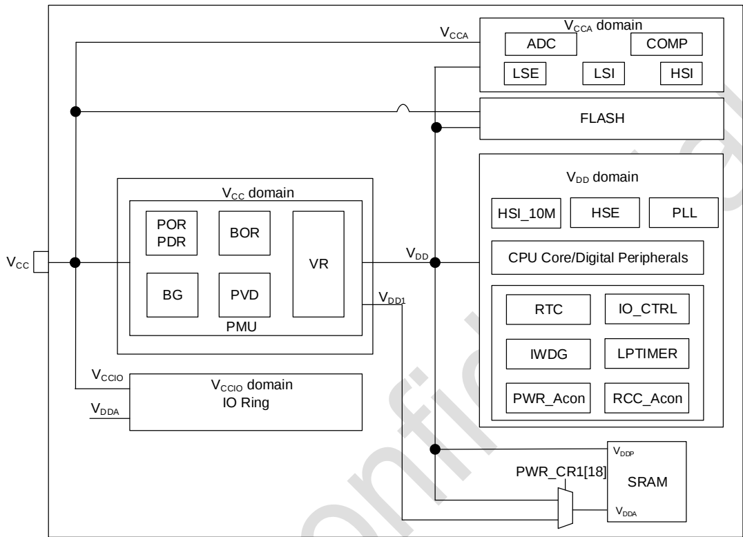
图 2-2 电源框图
