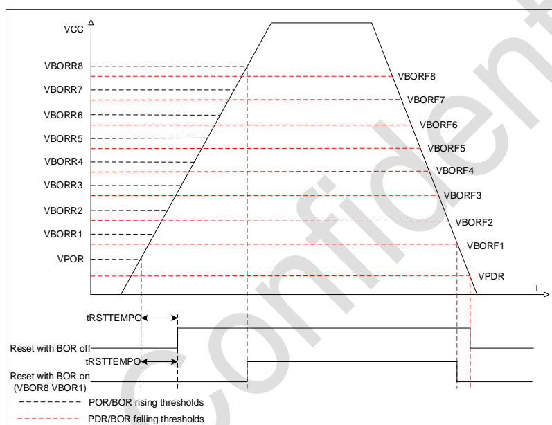
图 2-3 POR/PDR/BOR 阈值
