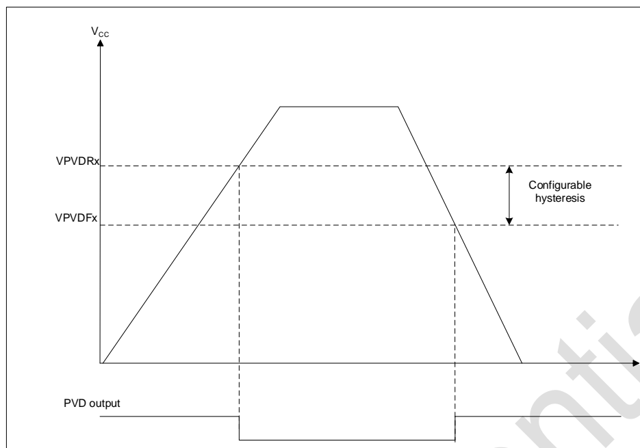
图 2-4 PVD 阈值
