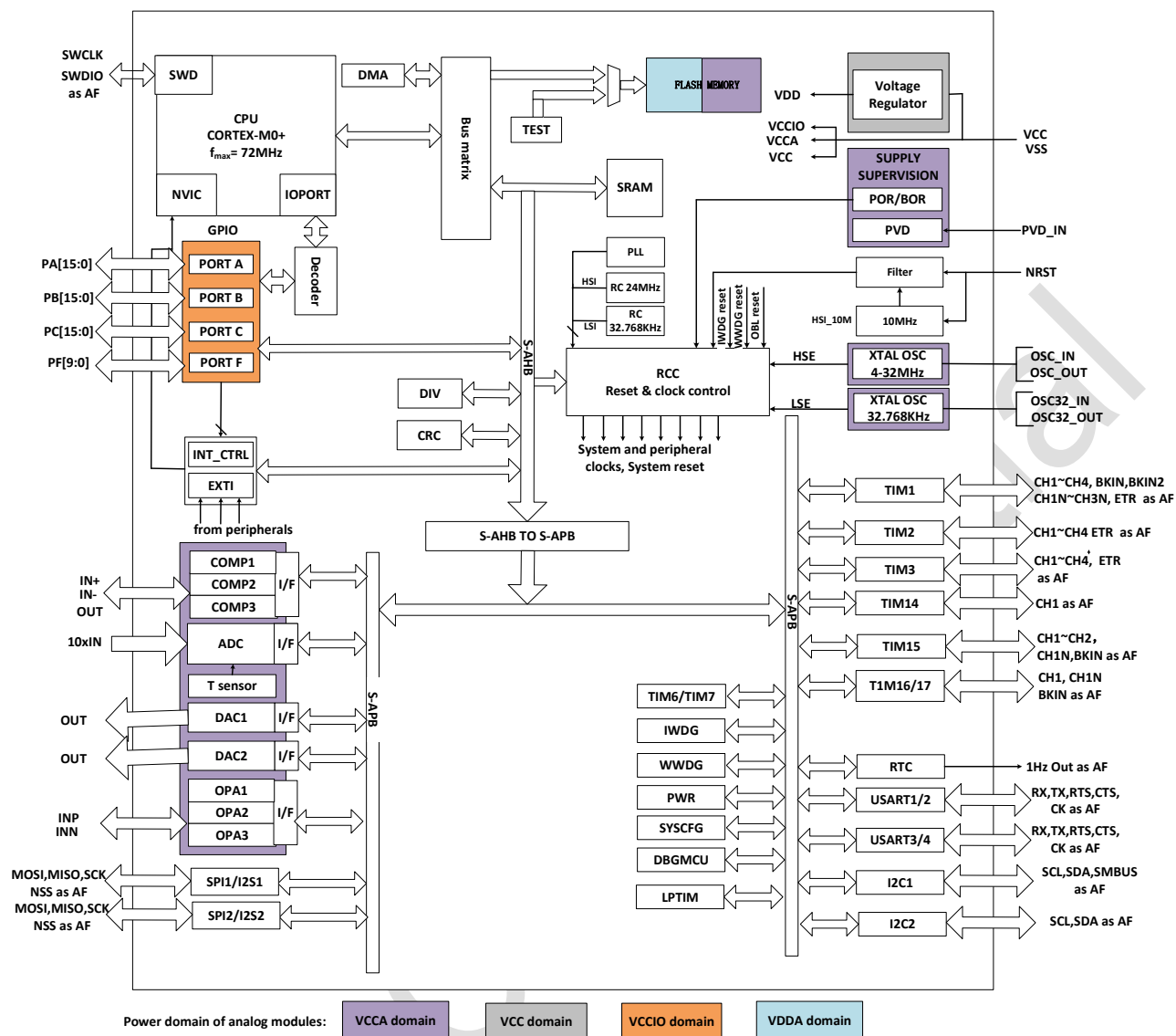
图 1-1 功能模块
