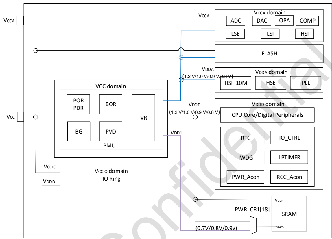
图 2-2 电源框图
