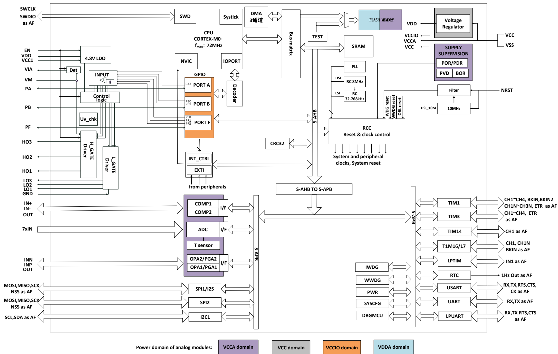
图 1-1 功能模块
