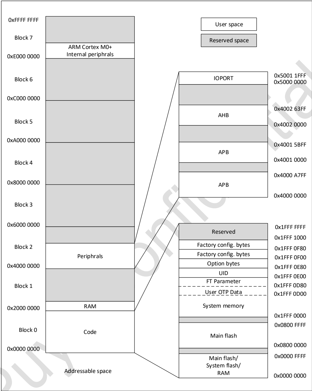
图 4-1 存储器映射
